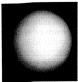
Uranus
