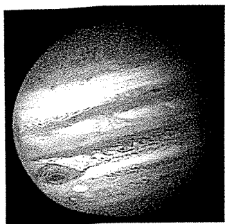
Jupiter
