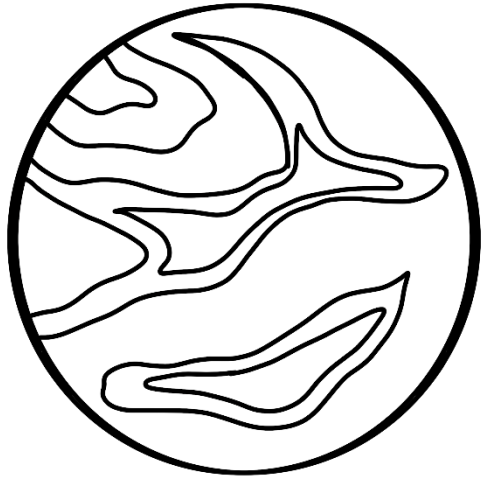
Venus
