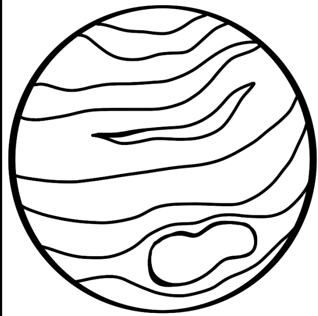
Jupiter
