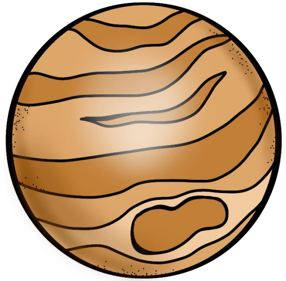
Jupiter
