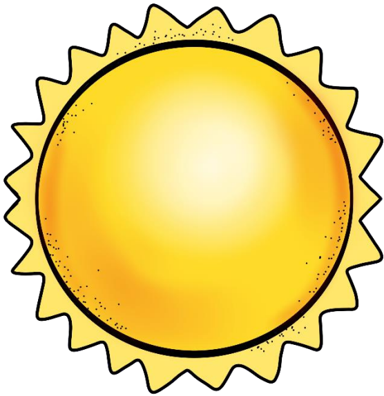
Sun
